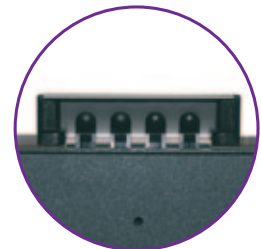
Von den vier verdeckten Tasten muß die richtige Kombination gedrückt werden. Dann läßt sich die Lade öffnen. Der erste Öffnungsversuch mit falscher Kombination aktiviert die Alarmklingel.
